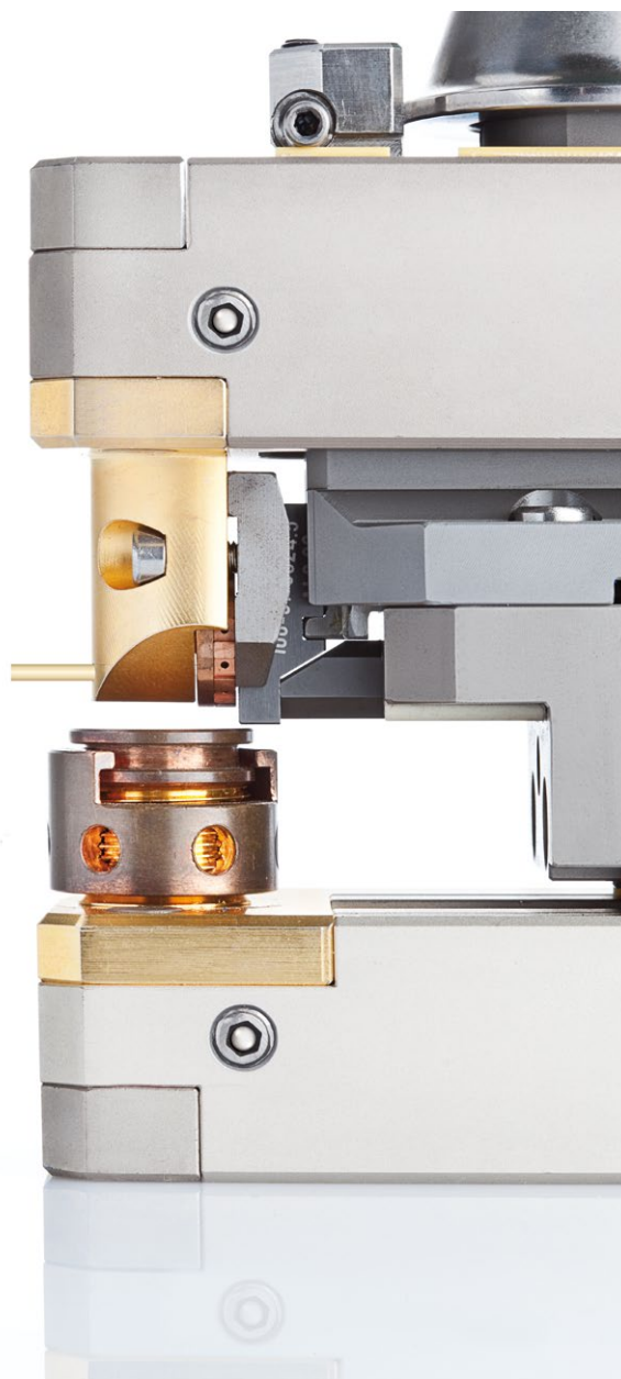
Corte de cuchilla con cinta de perfil
